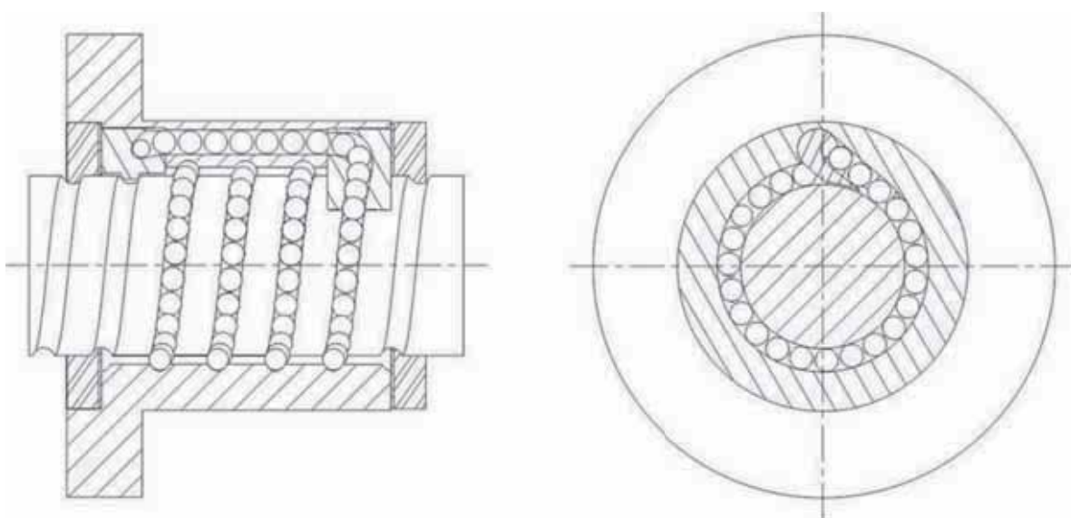
Fig. 3.23 S-type nut
